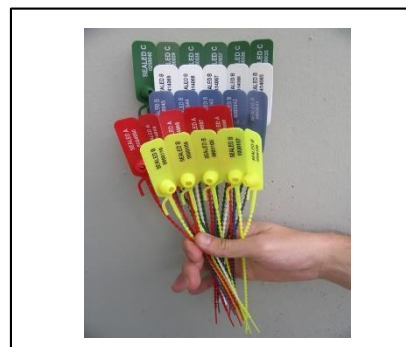
Art: JUPITER SEAL Kunststoffplombe mit Metallverschluss. Mit rundem Kabel Mit oder ohne Aufreissvorrichtung Hot Print Druck Dimensionen 2 x 315 mm 2 x 425 mm
