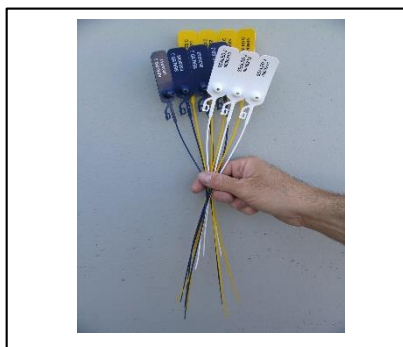
Art: JUPITER SEAL Kunststoffplombe mit Metallverschluss. Mit rundem Kabel Mit oder ohne Aufreissvorrichtung Hot Print Druck Dimensionen 3,3 x 315 mm 3,3 x 425 mm
