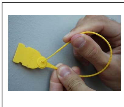
Art: SCITE SEAL LGH Kunststoffplombe mit Metallverschluss und rundem Kabel. Ohne Aufreissvorrichtung Laserdruck. Abmessungen 2x270 mm
