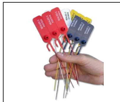
Art: JUPITER SEAL Kunststoffplombe mit Metallverschluss. Mit rundem Kabel Mit oder ohne Aufreissvorrichtung Hot Print Druck Dimensionen 1,3x 325 mm
